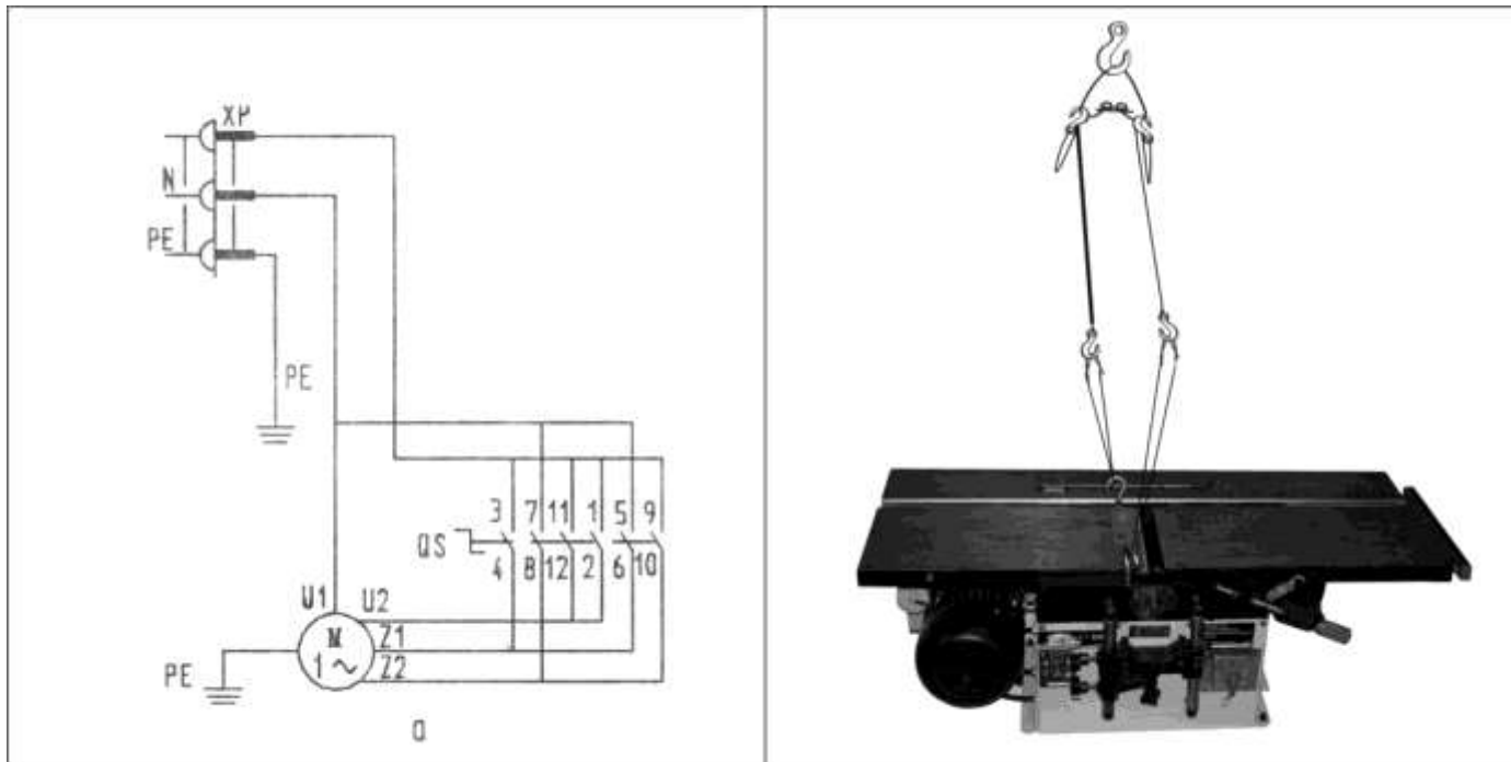
Электрическая схема
